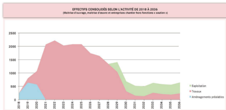
Figure 103 Effectifs consolidés selon l'activité de 2018 à 2036 (maîtrise d'ouvrage, maîtrises d'œuvre et entreprises chantier hors fonctions « soutien »)
