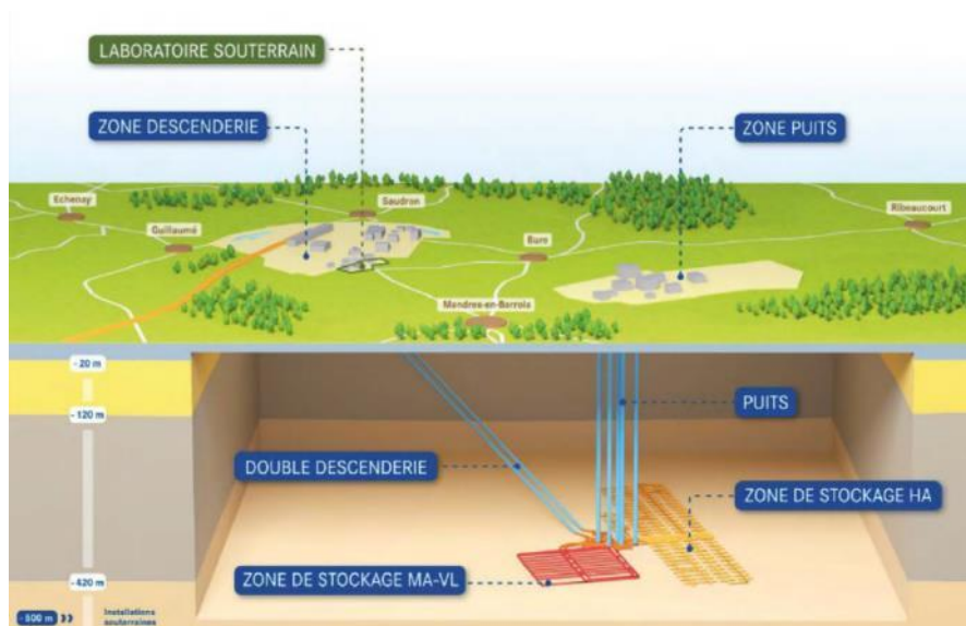
Vue en coupe du projet de centre de stockage Cigéo - Source : Ministère de la transition écologique et solidaire (janvier 2020).
